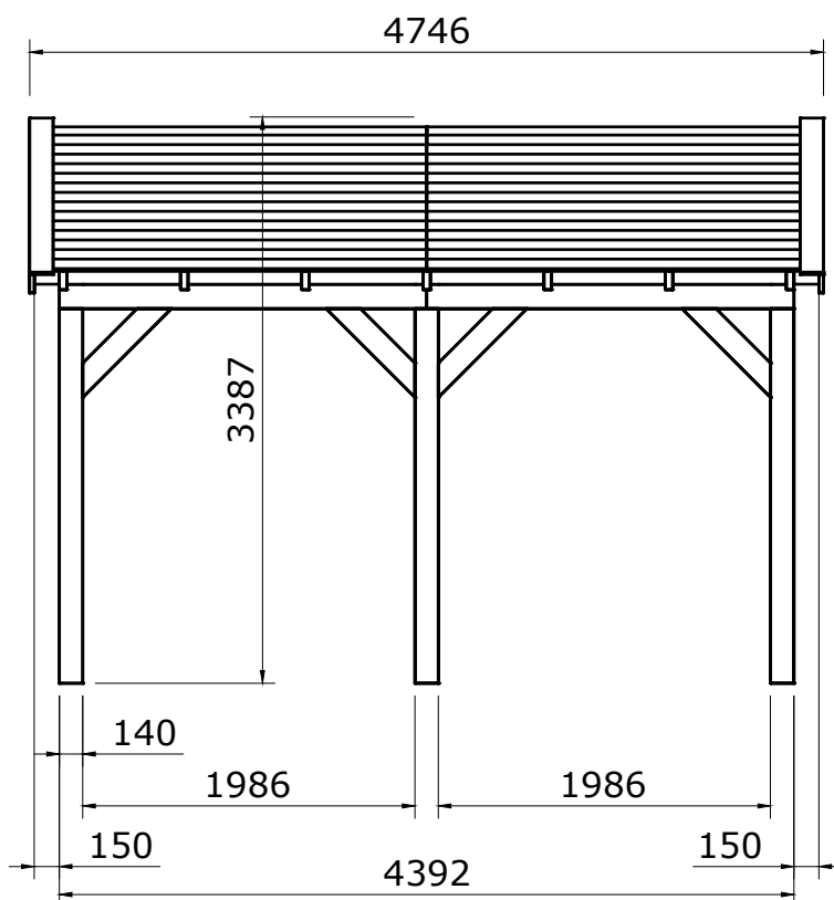
Vooraanzicht
