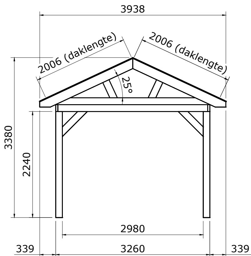
Rechter zijaanzicht
