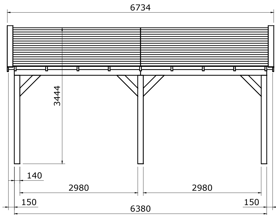
Vooraanzicht
