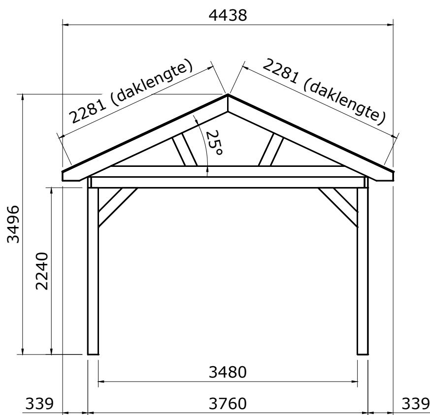
Rechter zijaanzicht
