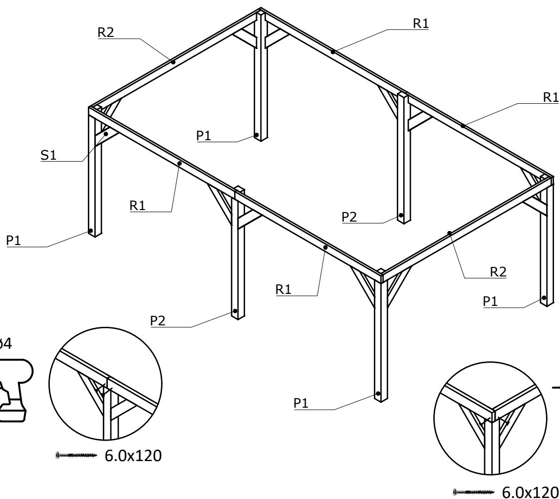
Bovenaanzicht
