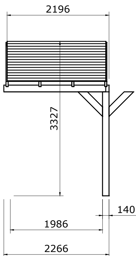
Vooraanzicht
