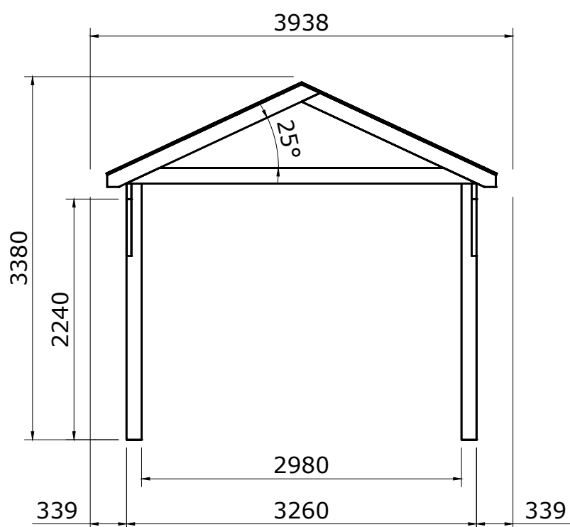
Rechter zijaanzicht
