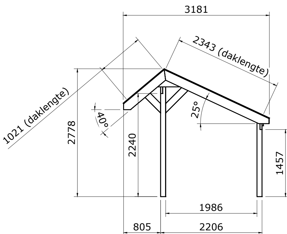
Rechter zijaanzicht
